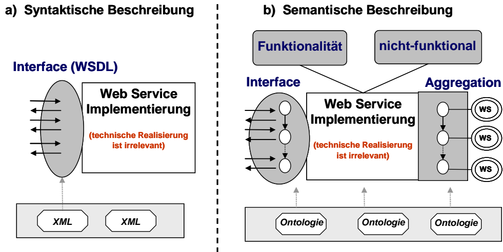
Abbildung 2: Von Syntaktischen zu Semantischen Web Service Beschreibungen
