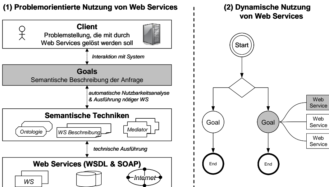
Abbildung 6: Der Goal-basierte Ansatz zur Unterstützung von Clients in SOA Systemen
