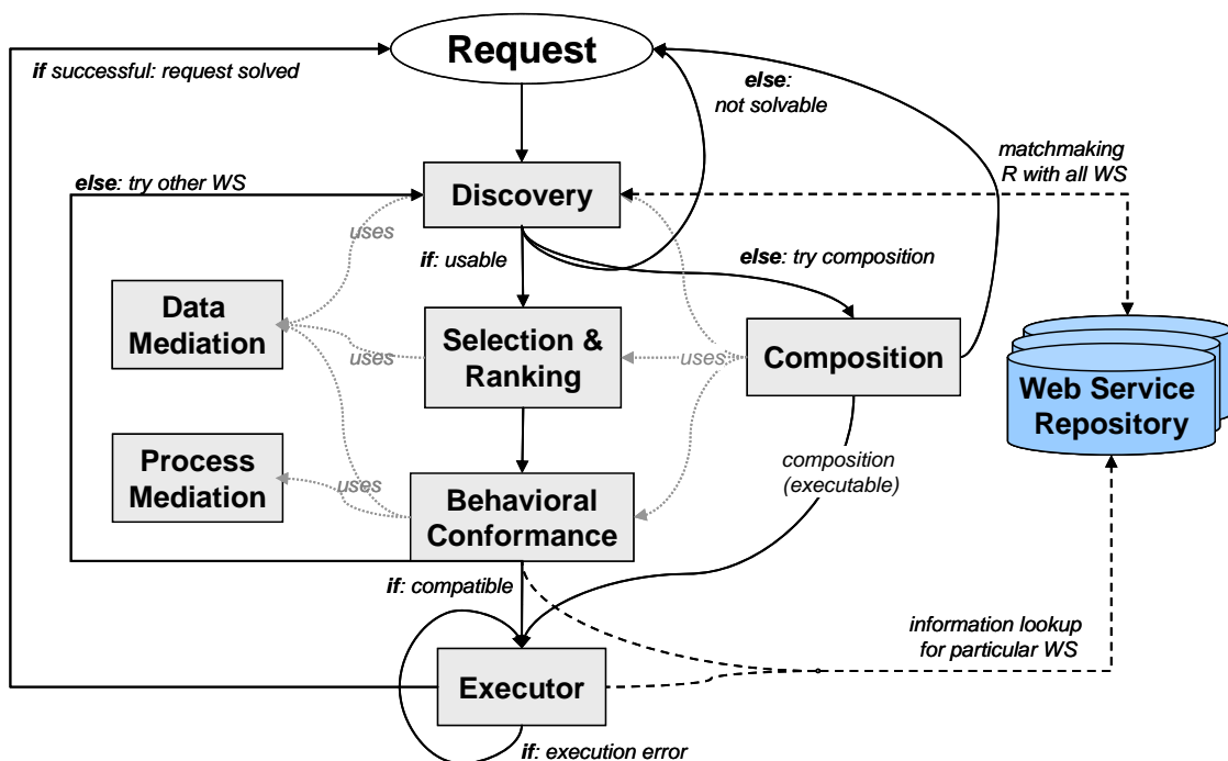
Abbildung 3: Automatisierter Web Service Nutzungszyklus
