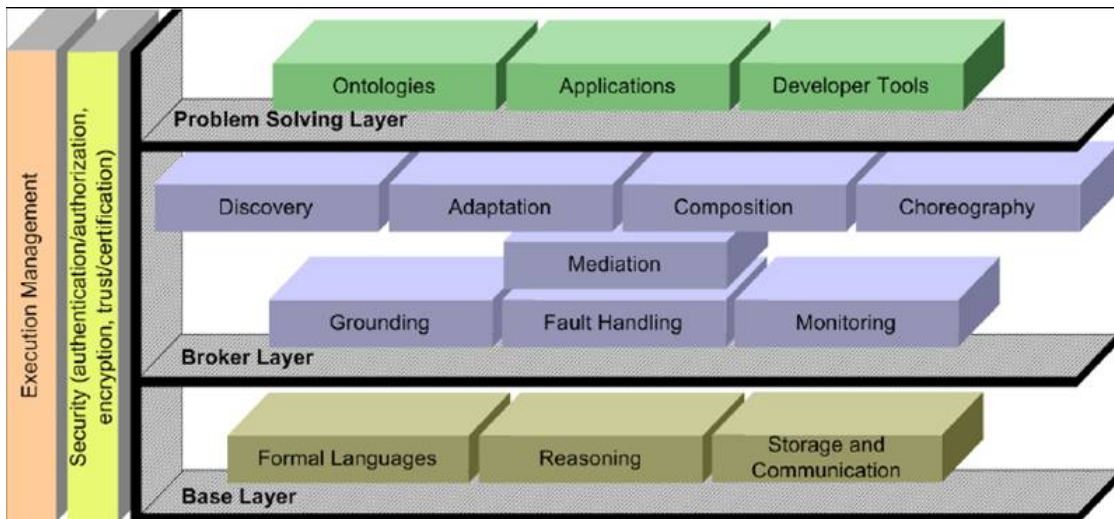
Abbildung 9: Überblick Web Service Execution Environment
