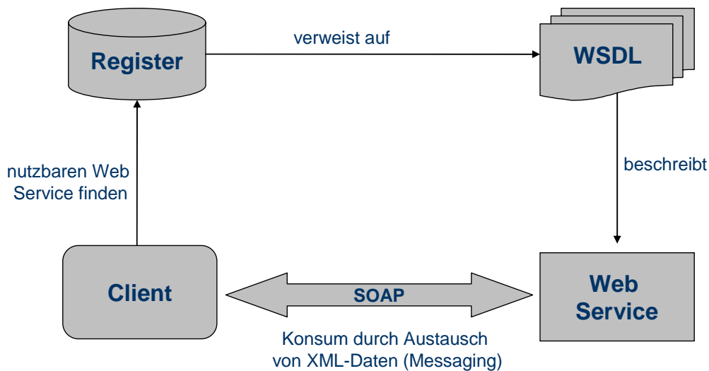
Abbildung 1: Web Service Nutzungszyklus
