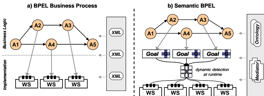
Abbildung 11: WSMO-basierte Erweiterung von BPEL
