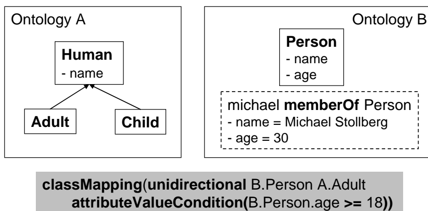
Abbildung 8: Beispiel zur ontologie-basierten Datenintegration
