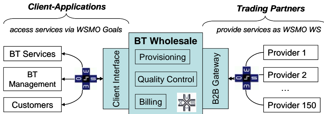
Abbildung 10: WSMO-basierte Telekom-Großhandelsplattform
